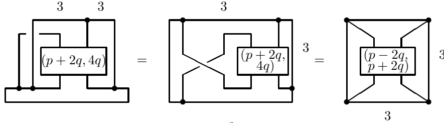
Рис. 2.5. Орбиболд ((6_2^3(p, q)/\langle \tau, \sigma \rangle)/\langle \rho \rangle)/\langle \lambda \rangle
