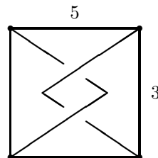
Рис. 0.1. Орбифолд наименьшего объема
